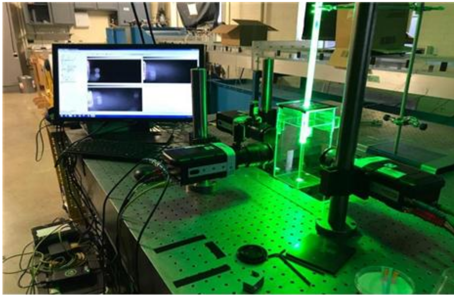
3차원 전자소자의 성능 측정을 위해 설치된 실험 장비
