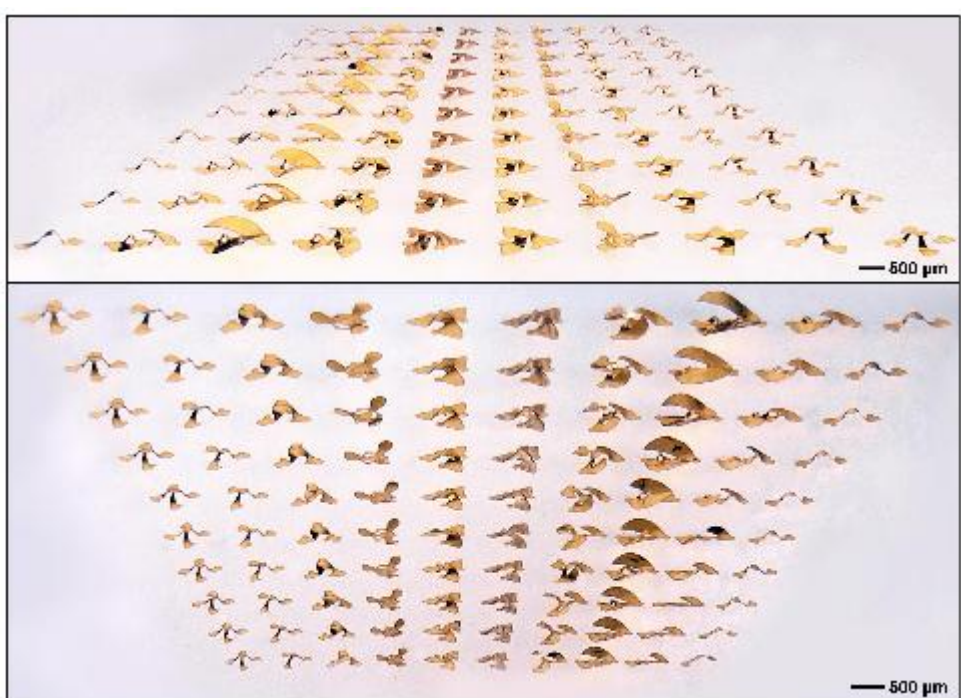
▲ 다양한 디자인과 크기를 갖는 3차원 전자소자.
